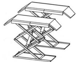
Saksinostin, jossa kuormauselimenä ovat lyhyet ajosillat.
