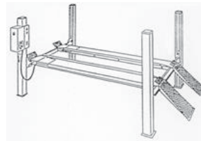
Nelipilarinostin, jossa kuormauselimenä ovat ajosillat.
