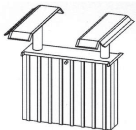
Kaksisylinterinostin, jossa kuormauselimenä ovat lyhyet ajosillat.
